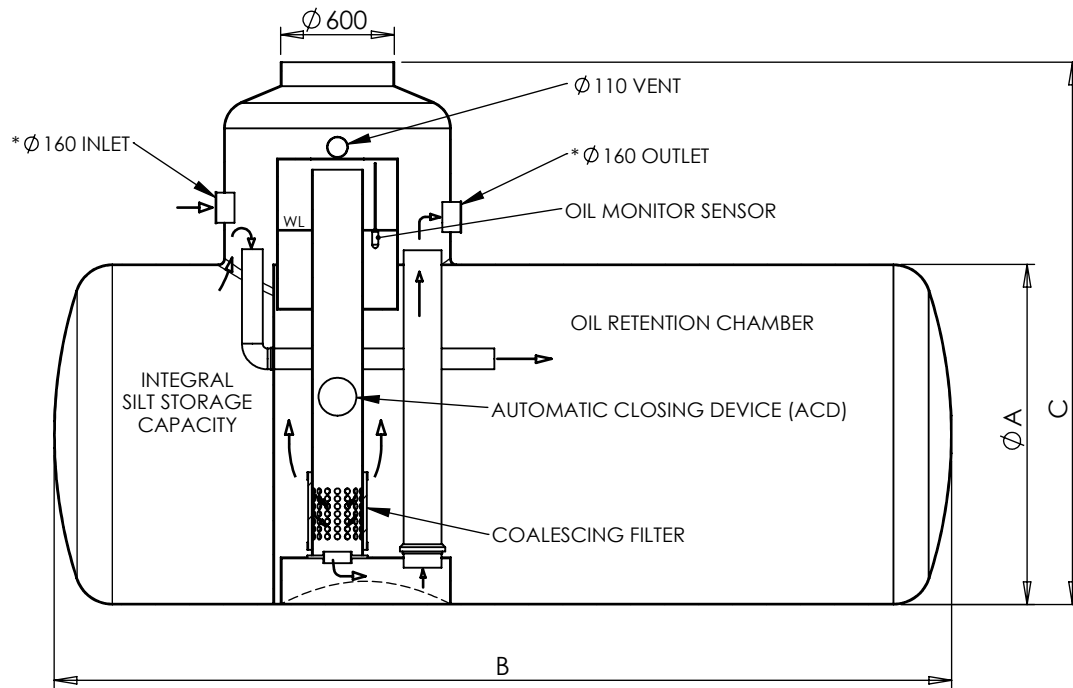
SECTION A-A SCALE 1 : 40
